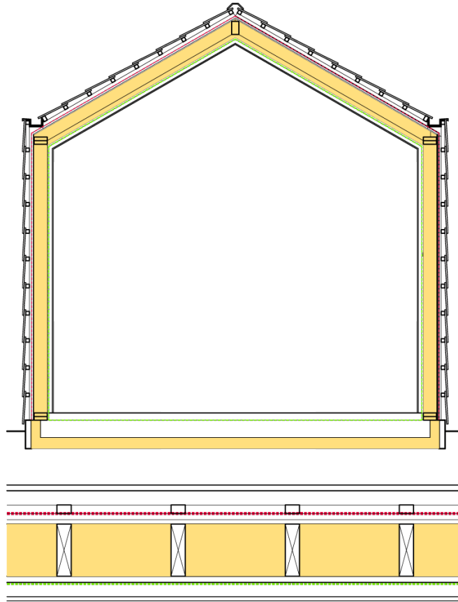
Casa Cachóns. Vivienda unifamiliar Passivhaus. Teo. A Coruña. Proyecto 2015. Obra 2018.
