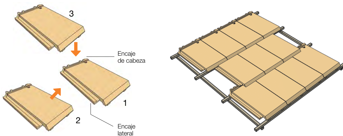
Figura 23. Encaje y solape de la teja plana lisa
