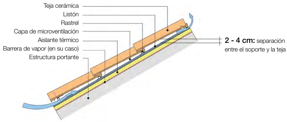
Figura 67. Recorrido del aire en la microventilación
