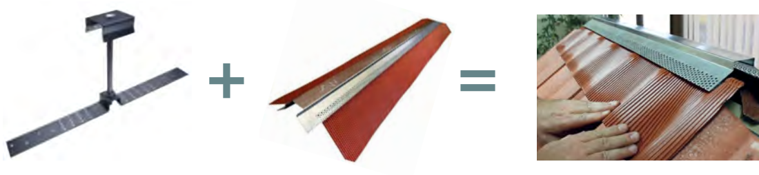
Figura 75. Soporte de caballete del tipo perfil metálico ranurado con forma de rastrel y sus componentes
