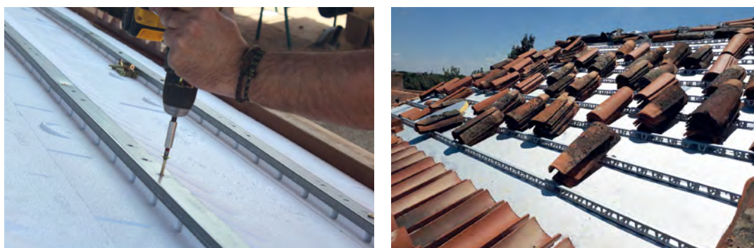
Figura 46. Rastreles simples sobre diferentes soportes continuos
