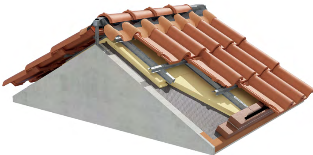
Figura 1. Nueva cubierta ventilada de teja cerámica
