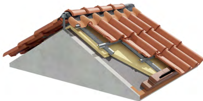
Figura 13. Cubierta con fijación en seco y con microventilación
