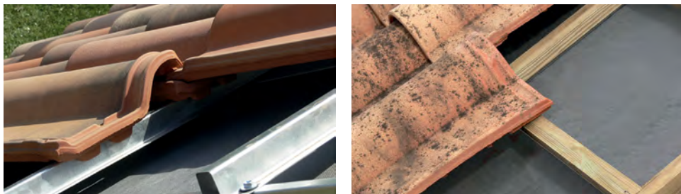
Figura 69. Espacio de circulación de la capa de microventilación de 4 cm por el doble rastrel
