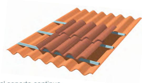
Figura 43. Rastreles fijados al soporte continuo
