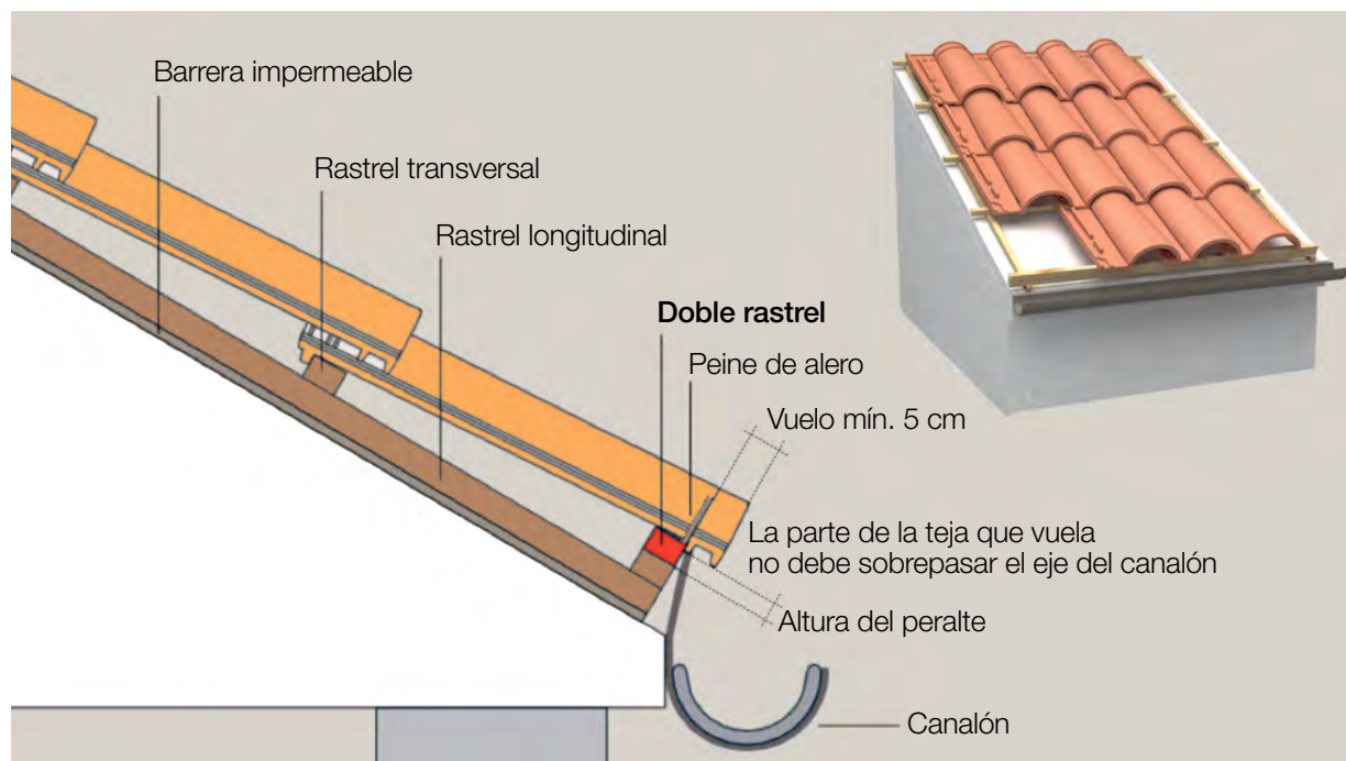
Figura 55. Esquema de colocación del doble rastrel en el alero
