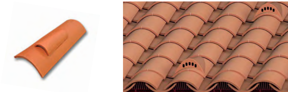
Figura 71. Cubierta con tejas de ventilación, por ser la distancia entre el alero y cumbre superior a 12 m
