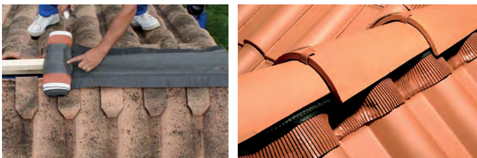
Figura 79. Cumbre con cuñas para caballete y sin ellas
